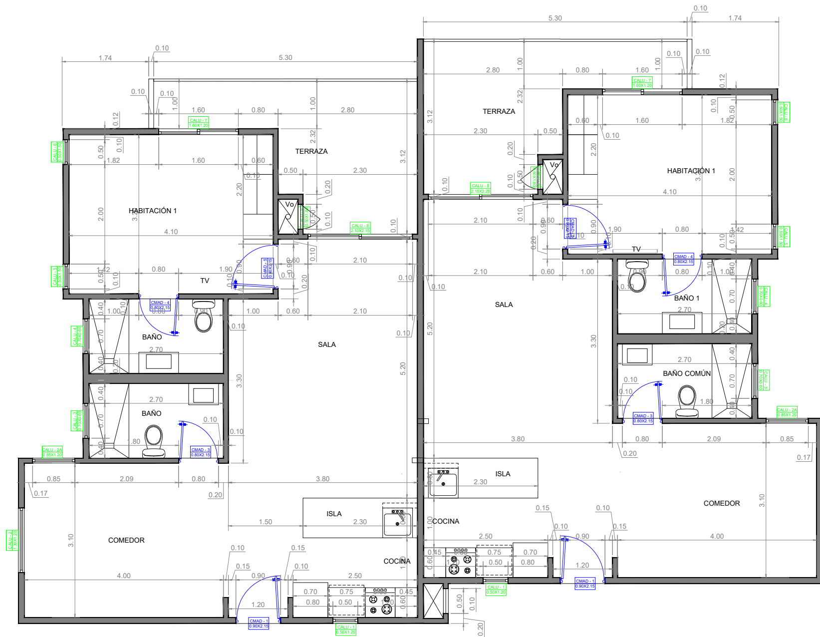
PLANO DIMENSIONADO
